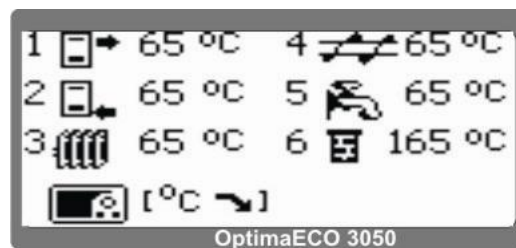
TEST CZUJNIKÓW
